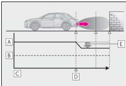
● 図 2（エンジン出力抑制制御時）
