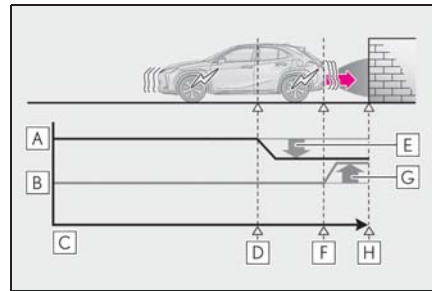
● 図 3（エンジン出力抑制制御かつブレーキ制御時）
